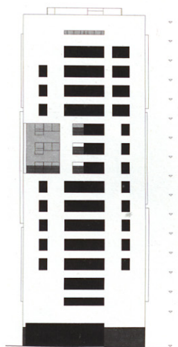
ALZADO TORRE
